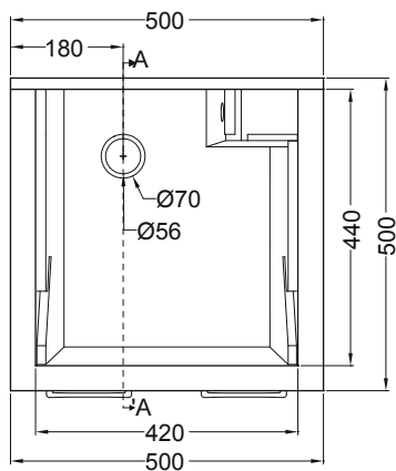
PIANTA
