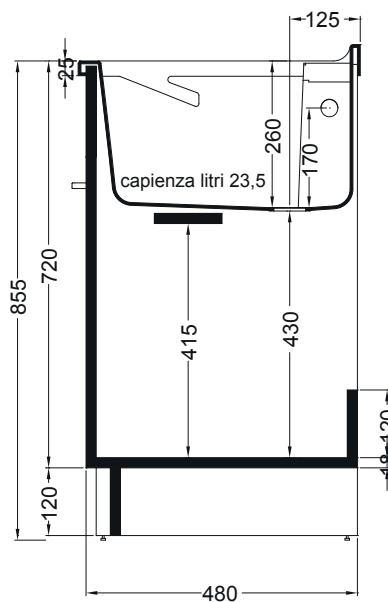
SEZIONE A-A'
