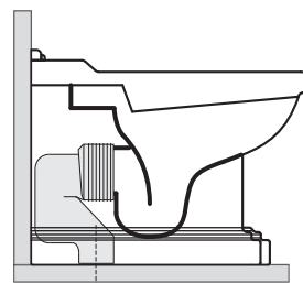
max. 180 // min. 150 con curva art. 13822
