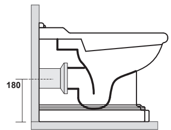
tubo di raccordo standard
