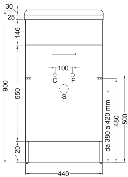
VISTA FRONTALE
