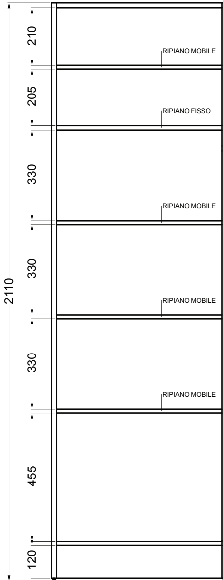
VISTA FRONTALE SENZA ANTE
