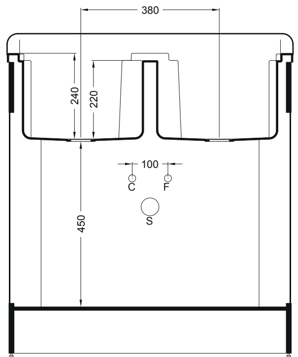
SEZIONE A-A'
