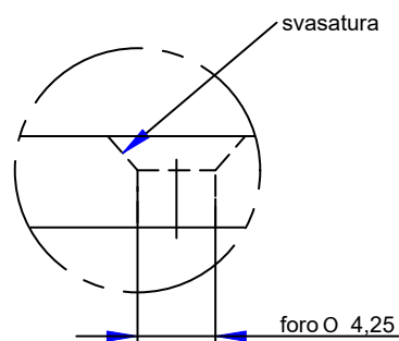
DETTAGLIO A
